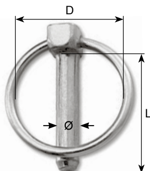
Goupille clips
